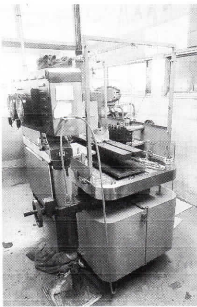
デンソー製ディーゼルポンプテストベンチ(CPS-21)
